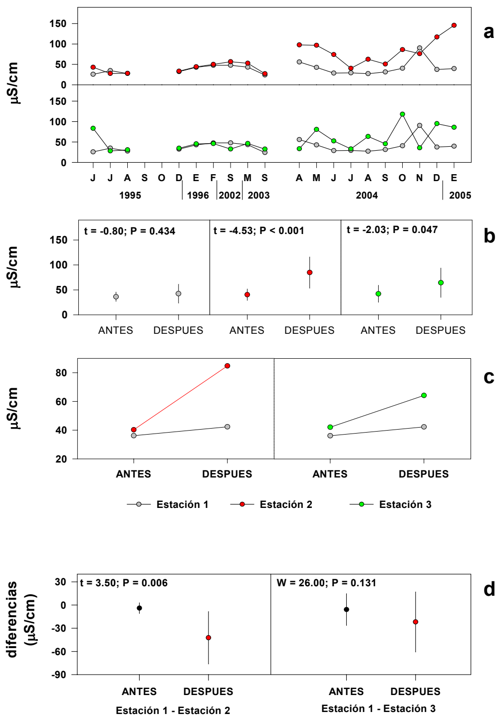
Figura 3. Conductividad del agua, a) variabilidad temporal de la Conductividad ( \mu\text{S/cm} ) en las estaciones 1, 2 y 3, b) resultados de los análisis estadísticos utilizados para comparar los datos de antes (1995-1996, 2002-2003) y después (2004-2005) en cada una de las estaciones de muestreo; los valores son promedios \pm 1 desviación estándar, c) comparación entre los valores promedios de las estaciones 1 y 2 y 1 y 3, d) resultados de los análisis estadísticos basados en las diferencias entre las estaciones 1 y 2 y 1 y 3; los valores son promedios de las diferencias \pm 1 desviación estándar.
